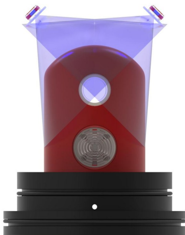
Fig. 4. Upper UV LEDs
